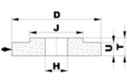
T38 MOLA CON MOZZO
