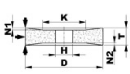
T21 DUE INCAVI SVASATI
