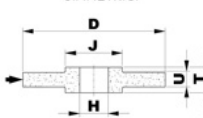
T39 MOLA CON DUE MOZZI SIMMETRICI
