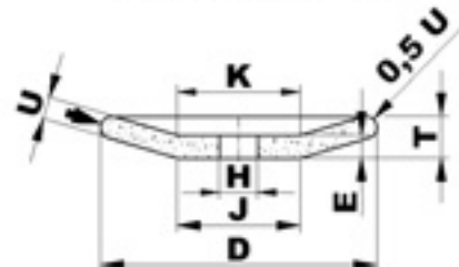
T13 MOLA A SCODELLA BORDO ARR. U=E
