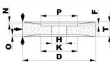
T25 INCAVO SVASATO SU INCAVO CILINDRICO INCAVO SVASATO SULLO LATO OPPOSTO
