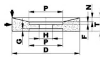
T24 INCAVO SVASATO SU INCAVO CILINDRICO ENTRAMBI SULLO STESSO LATO
