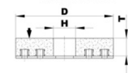
T36 MOLA FRONTALE CON INSERTI FILETTATI
