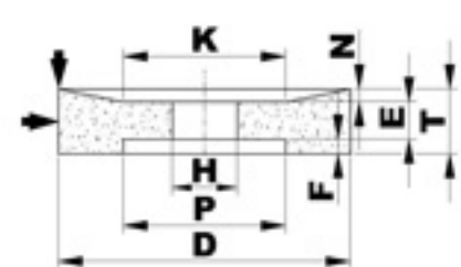
T22 UN INCAVO UN INCAVO SVASATO
