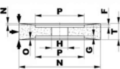
T26 INCAVO SVASATO SU INCAVO CILINDRICO SU ENTRAMBI I LATI
