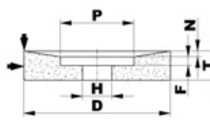
T23 INCAVO SVASATO SU INCAVO CILINDRICO ENTRAMBI SULLO STESSO LATO
