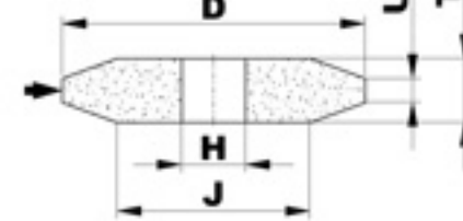
T4 MOLA A DOPPIO COLTELLO ( H < 0,67 \times D )
