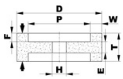
T8 MOLA A DOPPIA TAZZA
