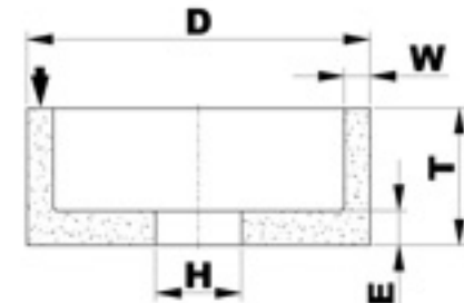
T6 TAZZA CILINDRICA
