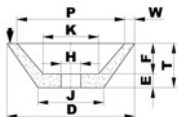
T11 MOLA A TAZZA CONICA
