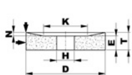
T20 UN INCAVO RASTREMATO
