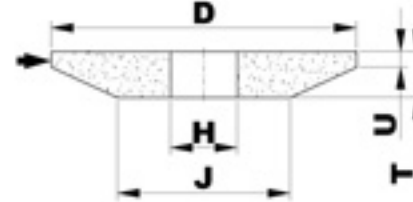
T3 MOLA A COLTELLO ( H < 0,67 \times D )
