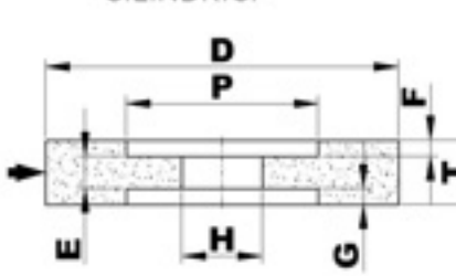
T7 MOLA CON DUE INCAVI CILINDRICI
