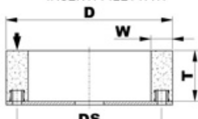
T37 MOLA AD ANELLO CON INSERTI FILETTATI
